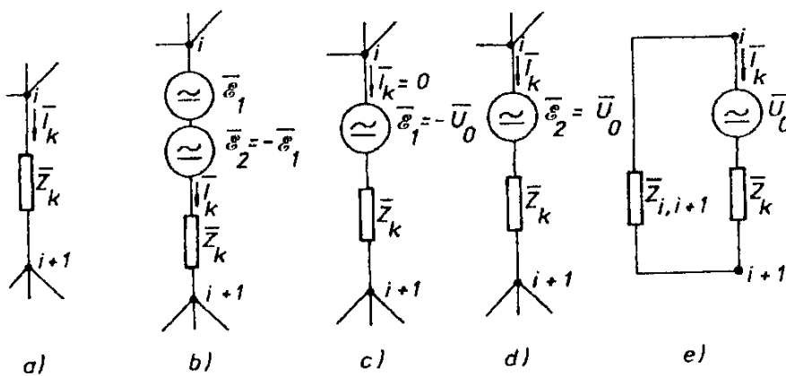
Obr. 8.12 K výkladu Théveninovy věty.
