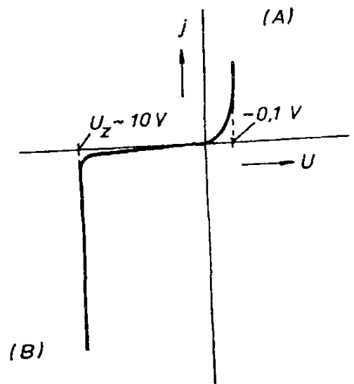
Obr. 7.28 Voltampérová charakteristika p-n přechodu (diody).
