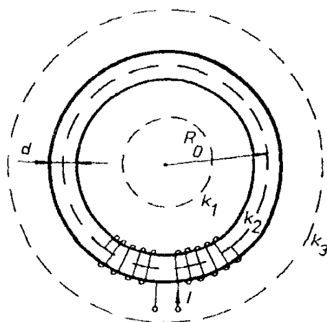
Obr. 3.22 Výpočet magnetické indukce toroidu.
