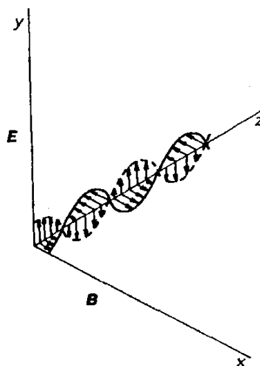
Obr. 5.3 Rozložení elektrického a magnetického pole v rovinné postupné vlně v zadaném okamžiku.
