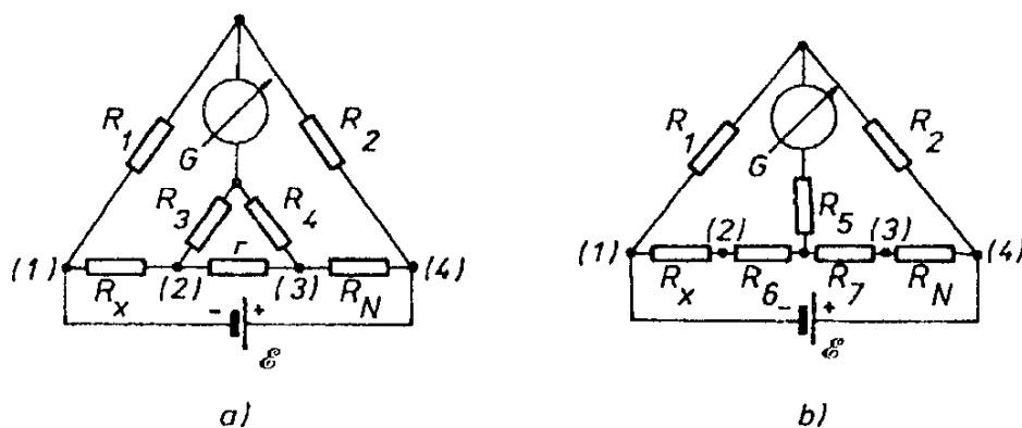
Obr. 8.19 K řešení rovnováhy Thomsonova dvojmostu: a) schéma Thomsonova dvojmostu, b) transformované schéma.
