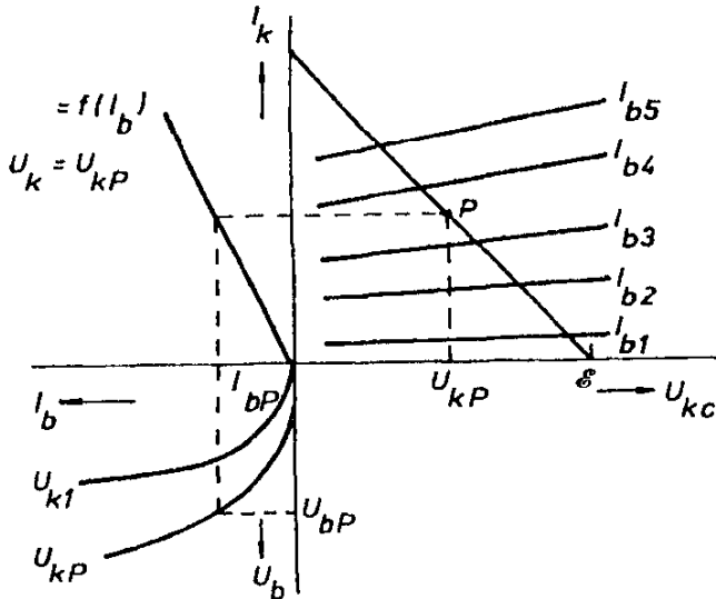
Obr. 8.30 Grafická metoda nalezení pracovního bodu tranzistoru.
