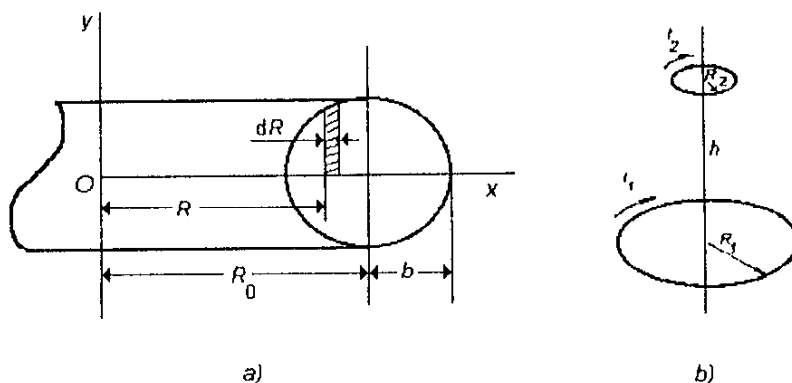
Obr. 4.10 K výpočtu a) vlastní indukčnosti toroidu, b) vzájemné indukčnosti dvojice sousých smyček.
