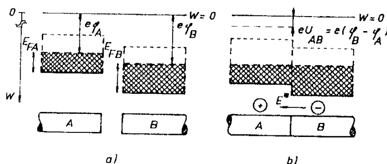
Obr. 7.25 K výkladu vzniku kontaktního napětí.
