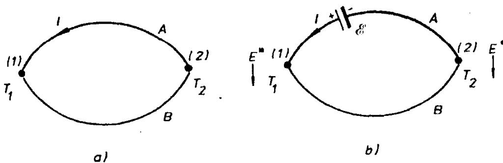
Obr. 7.23 K výkladu termoelektrických jevů: a) Seebeckův jev, b) Peltierův jev.
