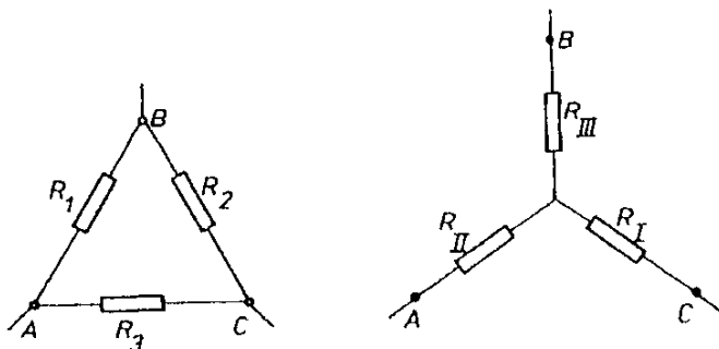
Obr. 3.13 Transformace hvězda trojúhelník.
