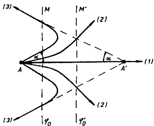
Obr. 6.8 Elektrostatické zrcadlo.
