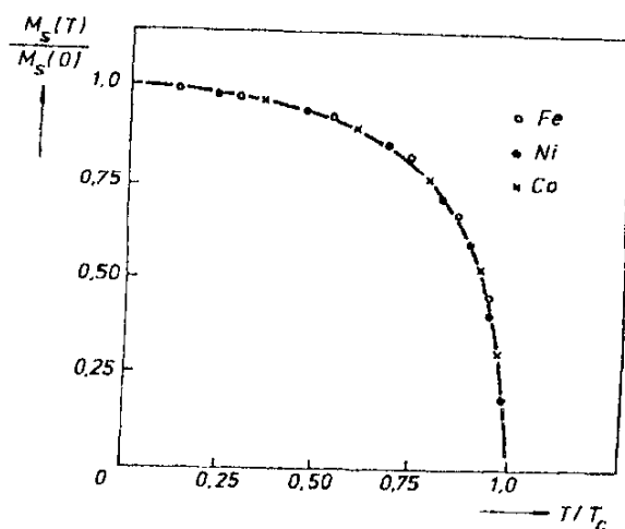
Obr. 7.15 Teplotní závislost spontánní magnetizace klasických feromagnetik Fe, Co, Ni.
