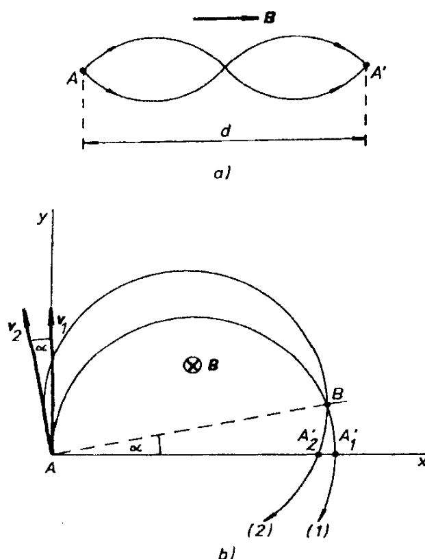
Obr. 6.11 Fokusace svazku nabitých částic magnetickým polem: a) podélné magnetické pole, b) příčné magnetické pole.
