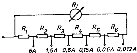
Obr. 8.32 Schéma Ayrtonova bočnicku k úloze Ú 8.3.
