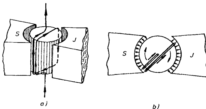
Obr. 4.24 Princip uspořádání magnetoelektrického měřicího přístroje.
