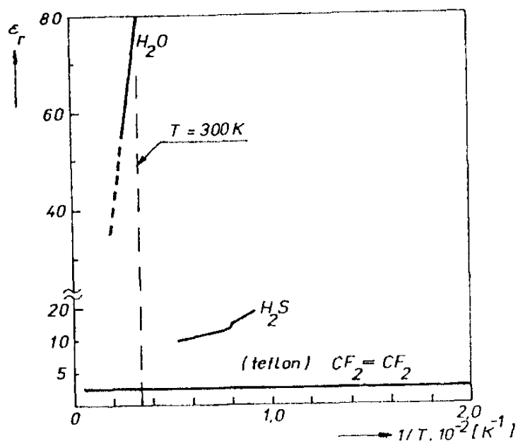
Obr. 7.9 Teplotní závislost permitivity některých látek.
