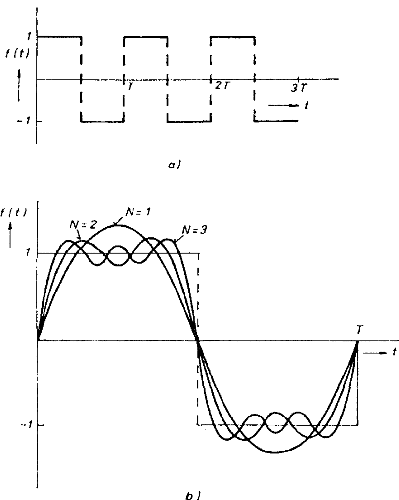
Obr. 8.21 a) Časový průběh „obdélníkové“ funkce, b) aproximace funkce z obr. 8.21a konečným počtem členů Fourierova rozvoje.
