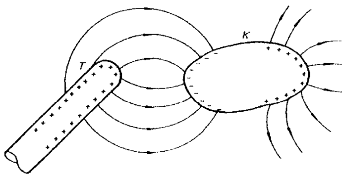
Obr. 1.43 Elektrostatická indukce.
