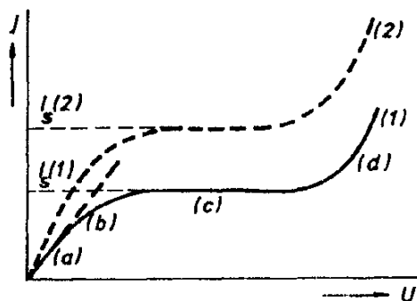
Obr. 7.41 Charakteristiky nesamostatného výboje v plynu.
