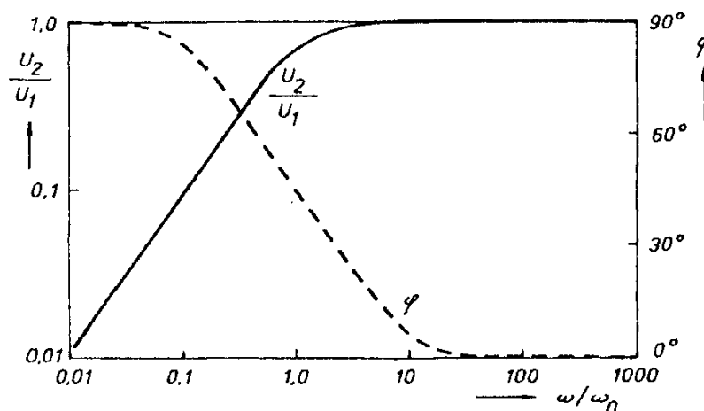
Obr. 8.23 Přenosová charakteristika čtyřpólu z obr. 8.22.
