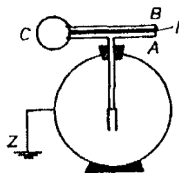
Obr. 7.21 Metoda detekce kontaktních napětí elektroskopem.
