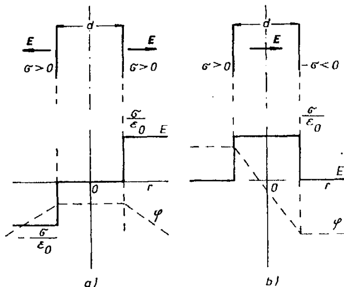
Obr. 1.20 Superpozice elektrostatických polí rovin nabitých: a) souhlasně, b) nesouhlasně.
