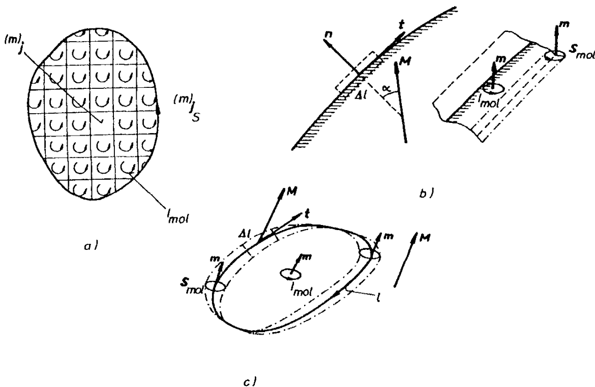
Obr. 3.28 K výkladu souvislosti magnetizačních proudů s nehomogenitou magnetizace.
