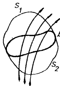
Obr. D 1.16 K určení toku solenoidálního vektorového pole uzavřenou plochou.
