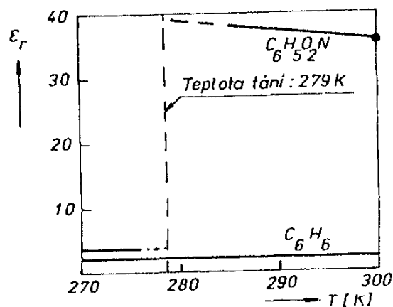
Obr. 7.8 Příklady teplotní závislosti relativní permitivity benzenu ( C_6H_6 ) a nitrobenzenu ( C_6H_5O_2N ) při přechodu z pevné fáze do kapalně fáze.
