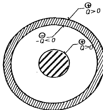
Obr. 1.46 Rozložení nábojů na povrchu koncentrických vodivých koulí.
