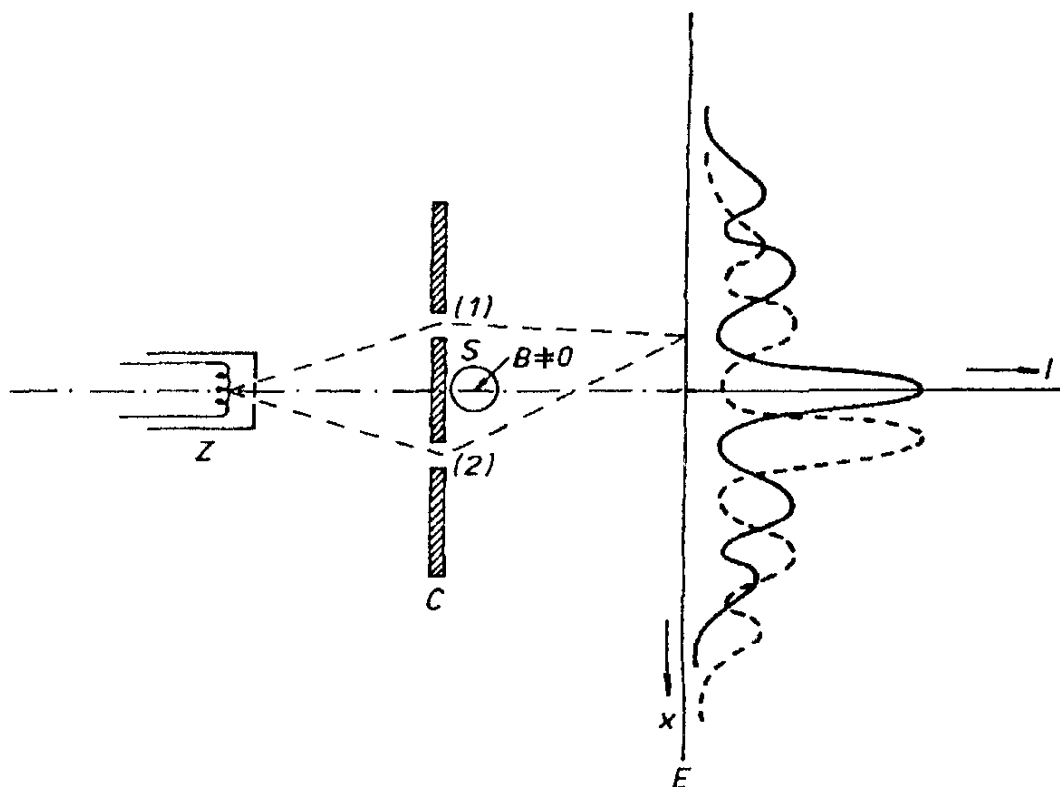
Obr. 6.1 K výkladu Bohmova–Aharonovova jevu.
