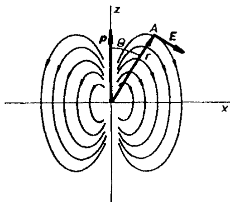
Obr. 1.28 Průběh siločar elektrostatičkého pole dipólu.
