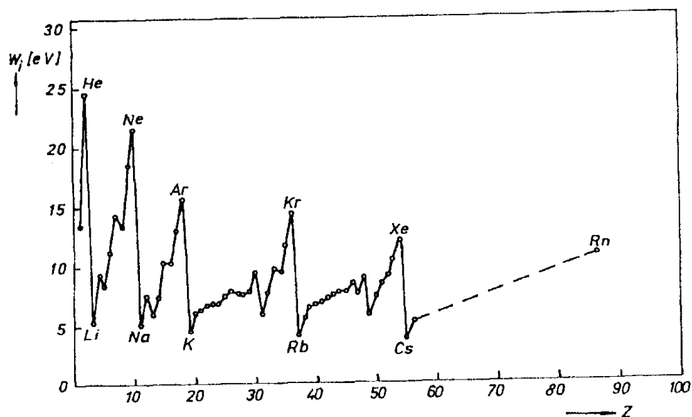
Obr. 7.3 Ionizační energie neutrálních atomů.
