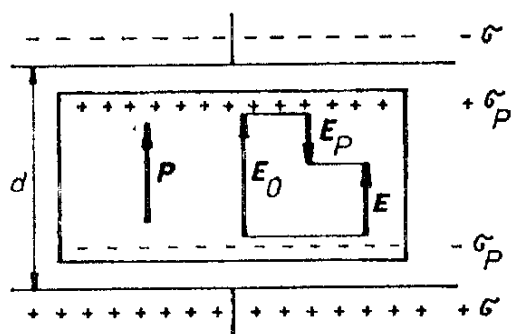
Obr. 1.62 Vliv dielektrika na elektrostatické pole mezi deskami kondenzátoru.
