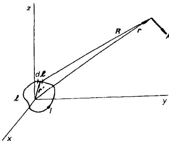
Obr. 3.23 K výpočtu vektorového potenciálu proudové smyčky.
