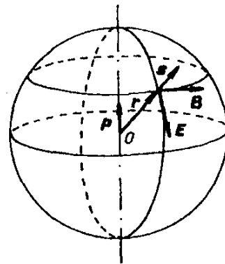
Obr. 5.4 Orientace elektrického a magnetického pole vůči směru šíření v kulové vlně.
