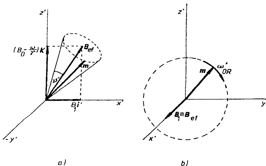
Obr. 6.17 K výkladu magnetické rezonance. Precese magnetického momentu v rotující soustavě souřadnic: a) mimo stav magnetické rezonance, b) ve stavu magnetické rezonance.
