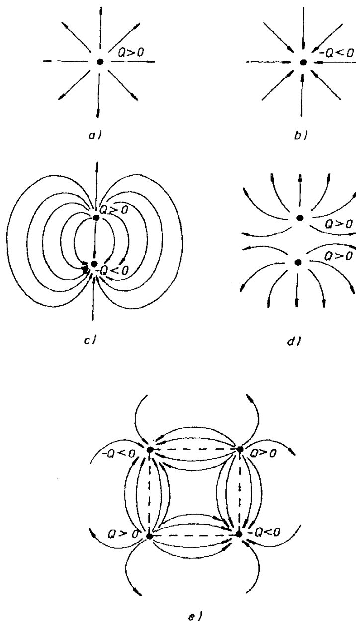
Obr. 1.9 Znázornění elektrického pole siločarami: a) kladného bodového náboje, b) záporného bodového náboje, c) konečného elektrického dipólu, d) soustavy dvou kladných bodových nábojů, e) konečného elektrického kvadrupólu.
