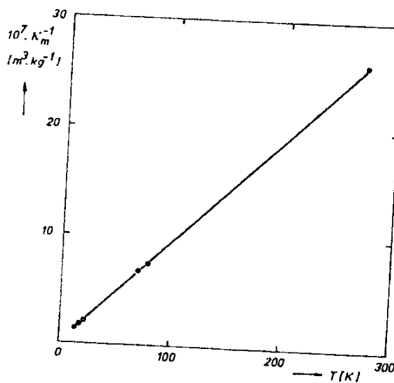
Obr. 7.12 Příklad teplotní závislosti magnetické susceptibility nekovového paramagnetika splňující Curieův zákon.
