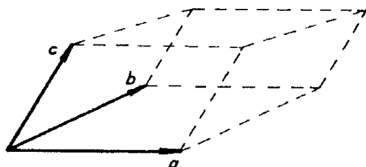
Obr. D 1.3 Geometrický význam smíšeného součinu tří vektorů.
