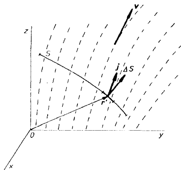
Obr. 3.1 K definici proudu a jeho hustoty.
