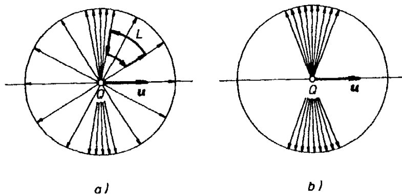
Obr. 2.4 Siločáry elektrického pole bodového: a) relativistického a b) ultrarelativistického náboje.
