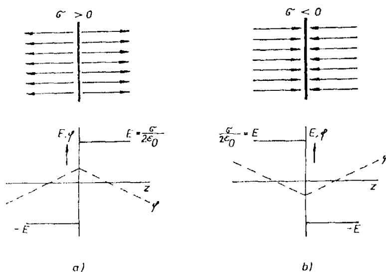
Obr. 1.19 Průběh elektrostatického pole roviny nabitě: a) kladným nábojem, b) záporným nábojem.
