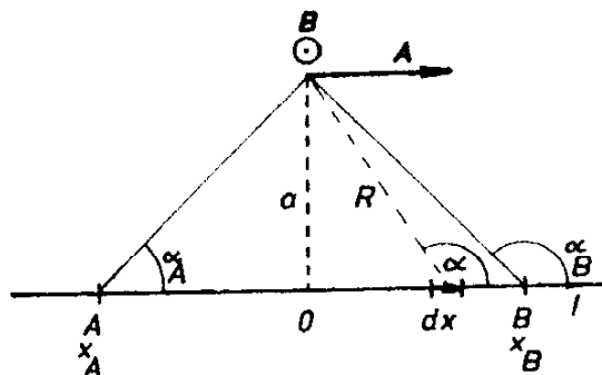
Obr. 3.19 Výpočet pole přímého vodiče pomocí Biotova–Savartova vzorce.
