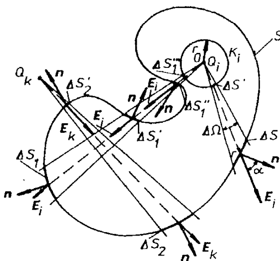
Obr. 1.11 K formulaci Gaussova zákona.
