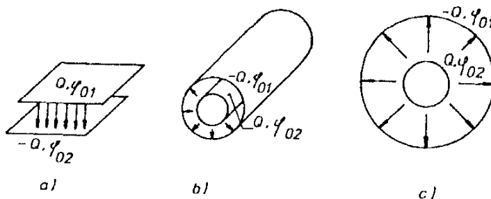
Obr. 1.53 Kondenzátory: a) deskový, b) válcový, c) kulový.
