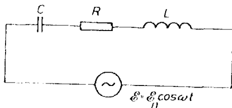
Obr. 4.20 Schéma sériového rezonančního obvodu.
