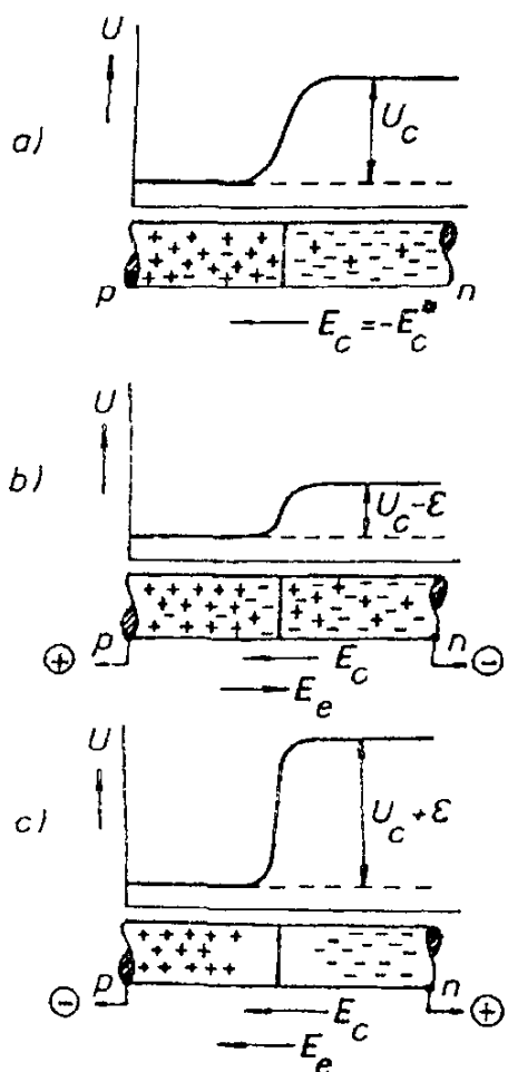
Obr. 7.27 Chování nositelů proudu v p - n přechodu: a) v nulovém elektrickém poli, b) ve vnějším elektrickém poli pólovaném v propustném směru, c) ve vnějším elektrickém poli pólovaném v nepropustném směru.
