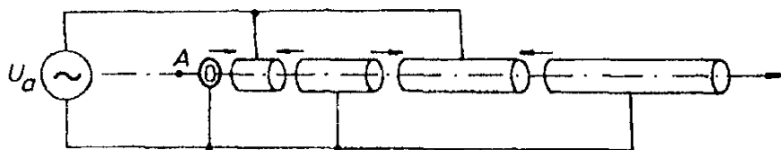
Obr. 6.13 Schéma lineárního urychlovače.
