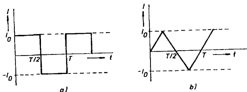
Obr. 8.38 Průběhy proudů pro výpočet středních a efektivních hodnot v úloze Ú 8.12: a) obdélníkový průběh, b) trojúhelníkový průběh.
