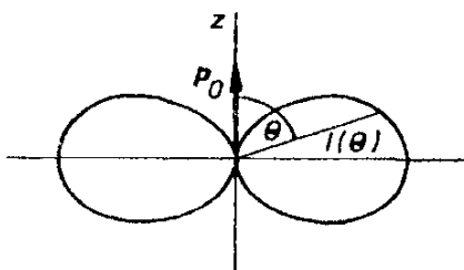
Obr. 5.5 Vyzařovací diagram lineárně polarizovaného dipólu.
