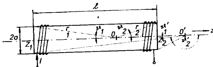
Obr. 3.21 Výpočet magnetické indukce na ose solenoidu.
