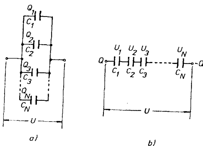
Obr. 1.55 Řazení kondenzátorů: a) paralelní, b) sériové.
