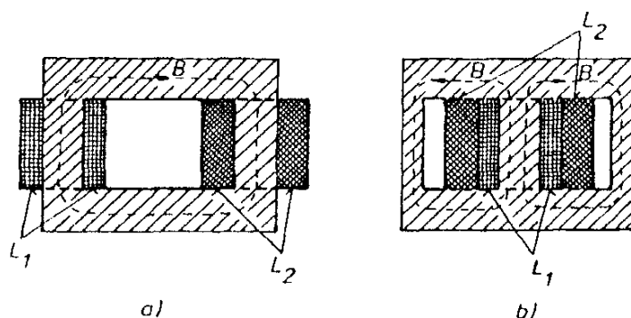
Obr. 4.17 Nejužívanější typy transformátorových jader.
