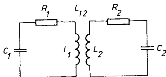
Obr. 4.22 Schéma indukčně vázaných rezonančních obvodů.
