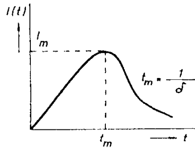
Obr. 4.14 Časová závislost proudu v aperiodickém stavu oscilačního obvodu.
