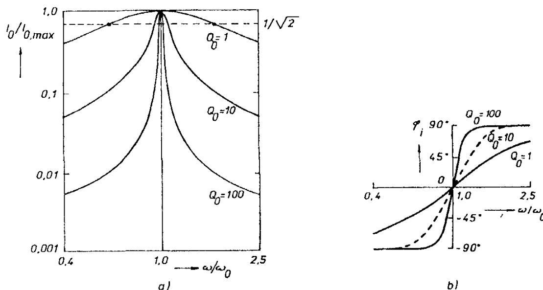
Obr. 4.21 Rezonanční křivky sériového rezonančního obvodu: a) redukovaná frekvenční závislost amplitudy napětí a proudu, b) redukovaná frekvenční závislost fázového úhlu.
