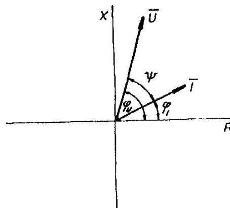
Obr. 8.4 Příklad fázového diagramu prvku s komplexní impedancí.
