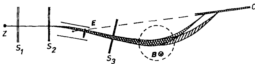
Obr. 6.15 Schéma Astonova hmotnostního spektrometru.
