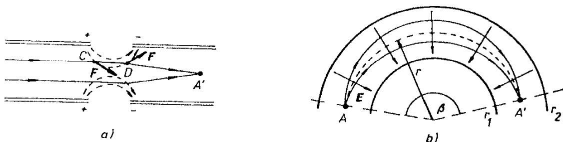
Obr. 6.10 Fokusace svazku nabitých částic elektrickým polem: a) podélné elektrické pole, b) příčné elektrické pole.
