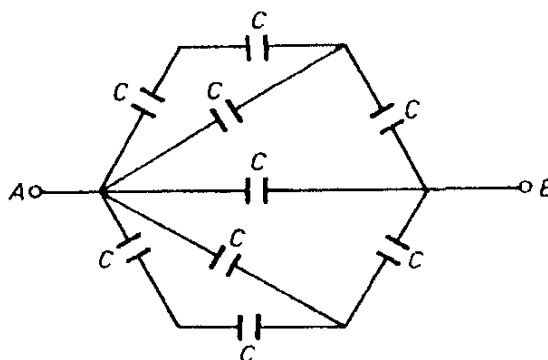
Obr. 1.66 Schéma zapojení kondenzátorů k úloze Ú 1.30.
