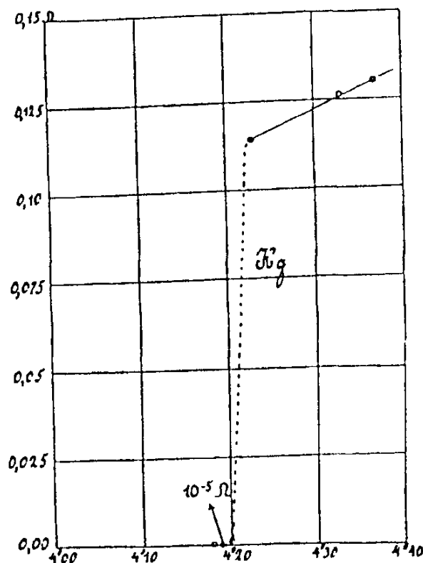
Obr. 7.31 Teplotní závislost elektrického odporu rtuti při přechodu do supravodivého stavu.
