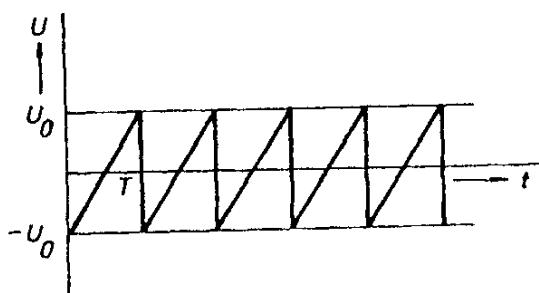
Obr. 8.39 Pilový průběh napětí pro výpočet efektivní hodnoty v úloze Ú 8.13.
