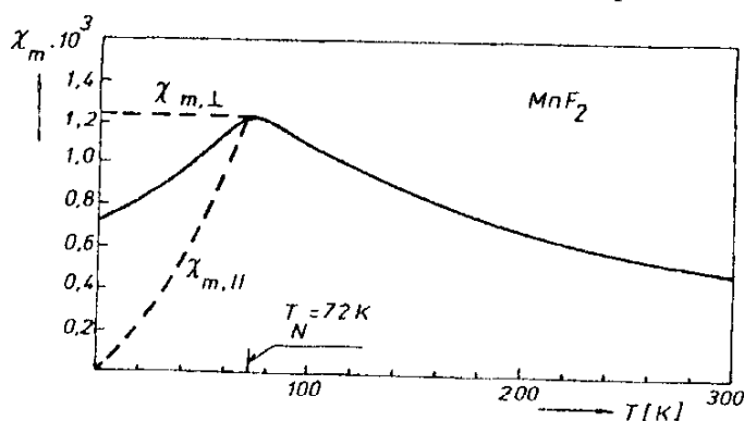
Obr. 7.14 Teplotní závislost magnetické susceptibility klasického antiferomagnetika \text{MnF}_2 .
