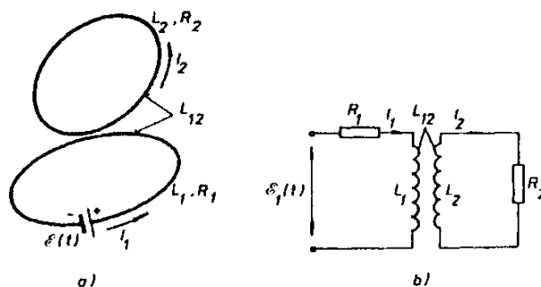
Obr. 4.16 a) indukčně vázané smyčky, b) schéma transformátoru.
