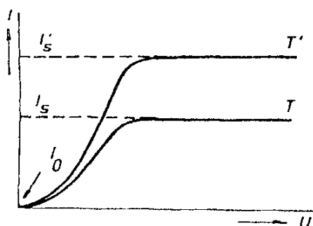
Obr. 7.35 Napětíová závislost emisního proudu při různých teplotách katody T' > T .
