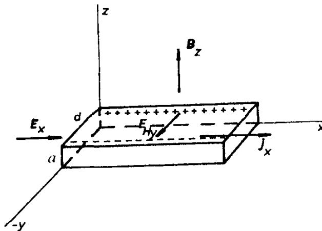
Obr. 7.18 Geometrická konfigurace studia Hallova jevu.
