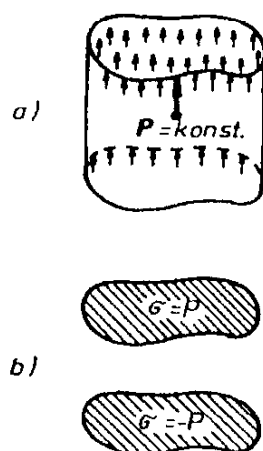
Obr. 1.37 a) Válec s homogenní objemovou polarizací, b) ekvivalentní rozložení plošných nábojů.
