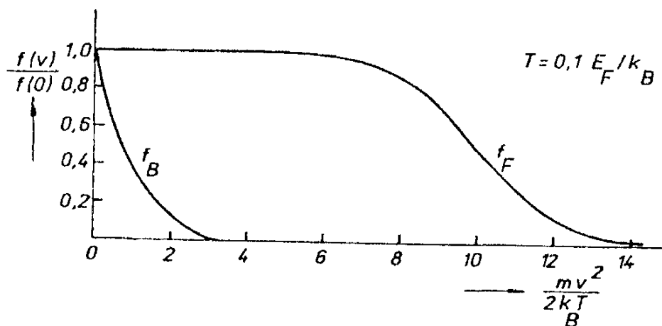
Obr. 7.7 Srovnání klasického a Fermiho–Diracova rozdělení.
