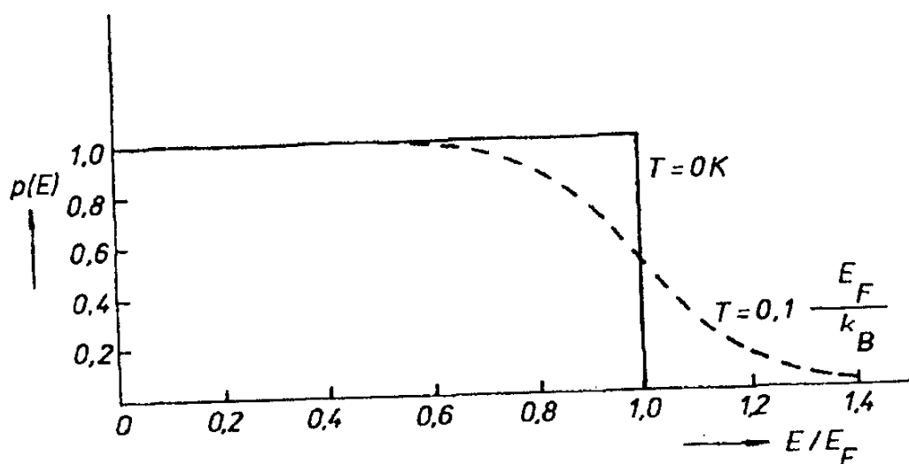
Obr. 7.6 Průběh Fermiho–Diracova rozdělení.
