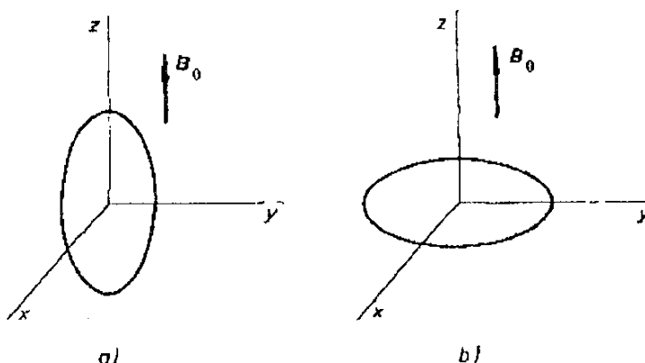
Obr. 3.34 K výkladu demagnetizačních polí v rotačním elipsoidu magnetovaném ve směru rotační osy z : a) protáhlý elipsoid, b) zploštělý elipsoid. V daném označení os platí pro hlavní hodnoty demagnetizačního faktoru N_1 = N_x , N_2 = N_y , N_3 = N_z .
