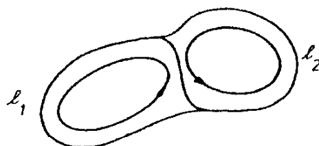
Obr. D 1.11 Sčítání cirkulací vektorového pole podél uzavřených křivek obepínajících dílčí plochy.
