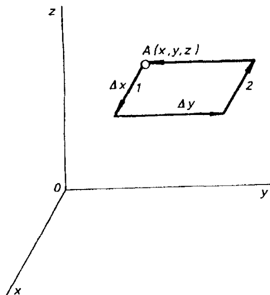
Obr. D 1.12 K odvození výrazu pro rotaci v kartézských souřadnicích.
