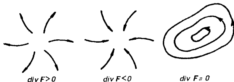
Obr. D 1.17 Kvalitativní průběh siločar vektorových polí: a) potenciální pole s kladným zdrojem, b) potenciální pole se záporným zdrojem, c) solenoidální pole.
