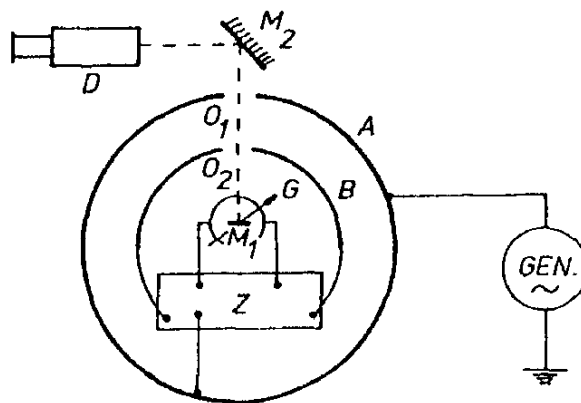
Obr. 1.49 Kvazistatická metoda měření elektrostatického pole uvnitř duté nabitě koule.
