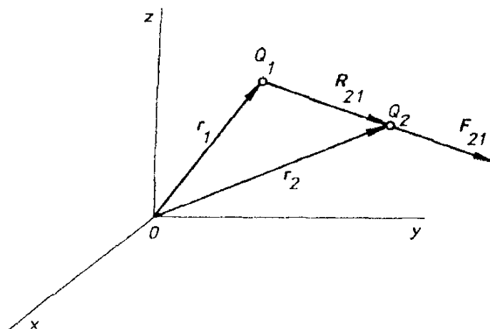
Obr. 1.1 K vzájemnému silovému působení dvou bodových nábojů.
