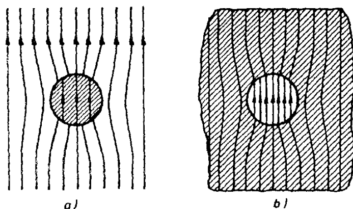
Obr. 1.64 Kvalitativní průběh elektrostatického pole: a) v okolí dielektrické koule, b) v okolí dutiny v dielektriku.
