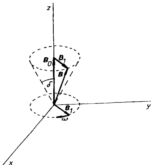
Obr. 6.16 K výkladu magnetické rezonance. Precese výsledného magnetického pole v laboratorní soustavě souřadnic.
