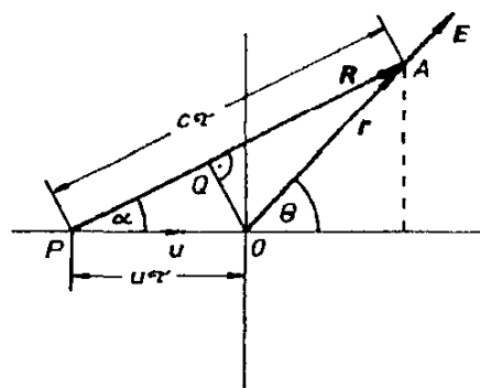
Obr. 2.5 K odvození intenzity elektrického pole bodového pohybujícího se náboje se zřetelem ke konečné rychlosti šíření signálu.
