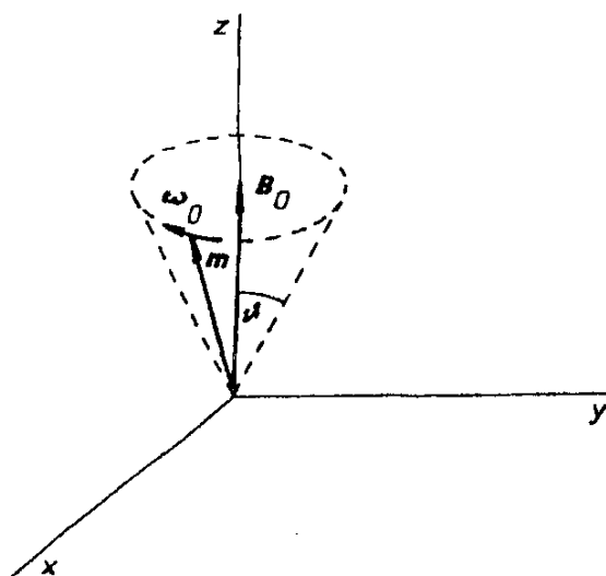
Obr. 6.7 Larmorova precese magnetického momentu \mathbf{m} .
