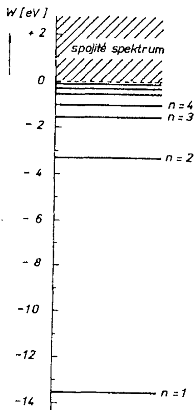
Obr. 7.1 Zjednodušené schéma energetických hladin atomu vodíku.
