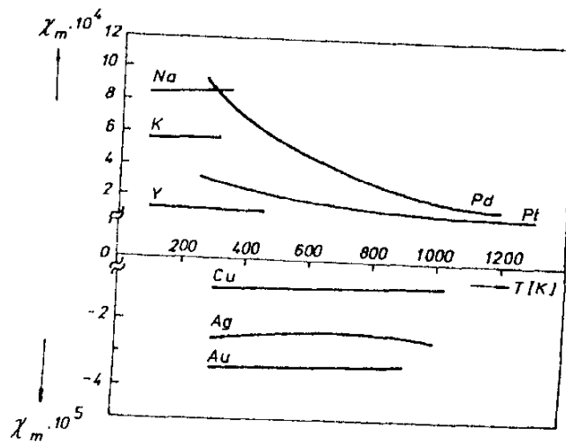
Obr. 7.11 Příklady teplotní závislosti magnetické susceptibility paramagnetických a diamagnetických kovů
