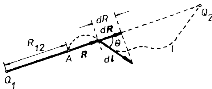
Obr. 1.4 K odvození energie soustavy dvou bodových nábojů.
