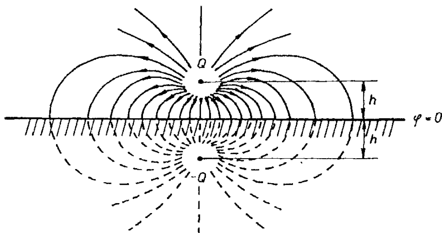
Obr. 1.57 K metodě elektrostatického zobrazení.
