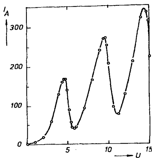
Obr. 7.44 Závislost proudu na urychlovacím napětí ve Franckově–Hertzově experimentu pro případ rtuti.
