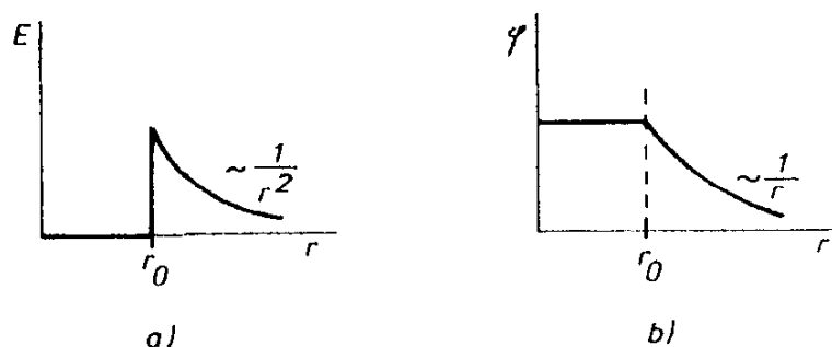
Obr. 1.22 Elektrostatičké pole nabité kulové slupky: a) průběh intenzity, b) průběh potenciálu.
