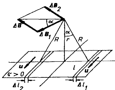
Obr. 2.9 K odvození magnetické indukce plošného rovinného proudu.
