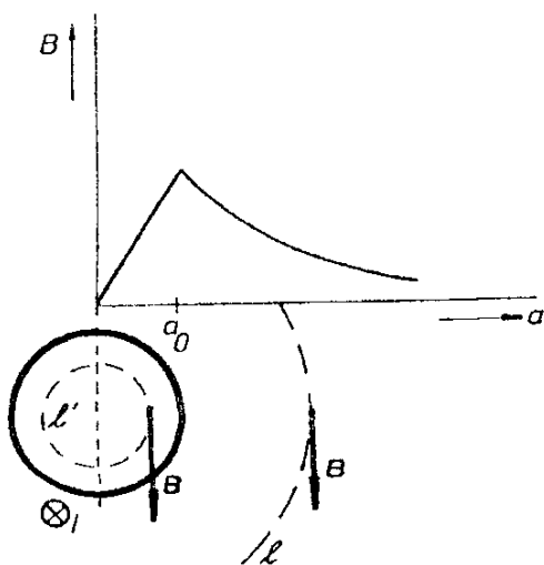
Obr. 3.18 Průběh magnetické indukce nekonečně dlouhého přímého vodiče.
