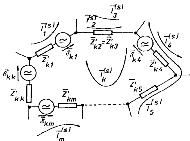
Obr. 8.10 K výkladu metody smyčkových proudů.
