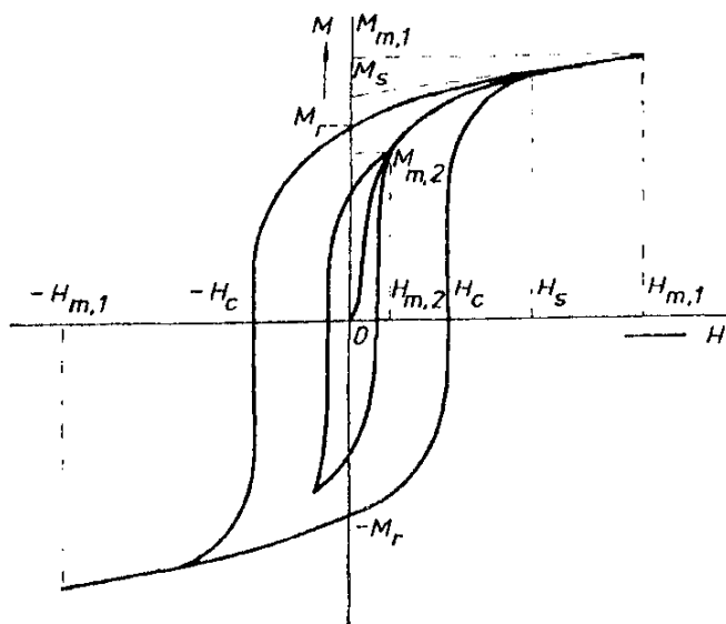
Obr. 3.29 Hysterezní smyčka feromagnetika.
