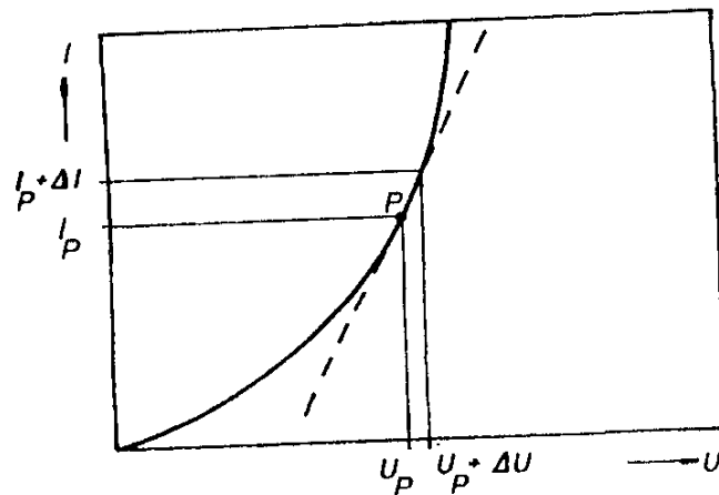
Obr. 8.2 K výkladu dynamického odporu dvojpólu.
