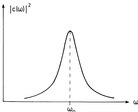
Fig. 16.10. Lorentzian line
